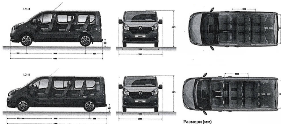
Размери (мм)
